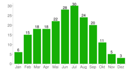
Ertragsverteilung über ein Jahr [kWh/Monat und m2]:
